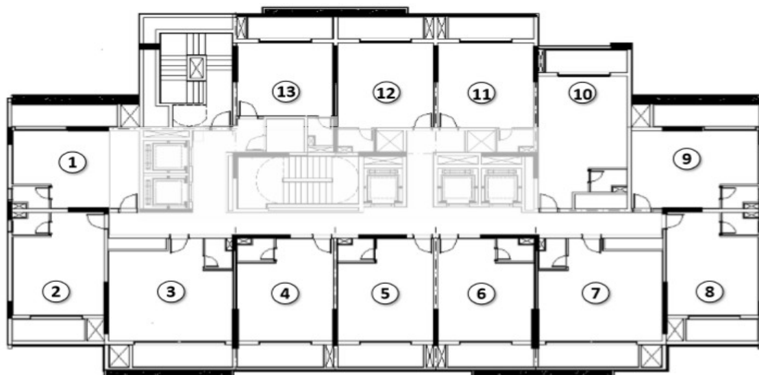
1º AO 3º PAVIMENTO - COMERCIAL
