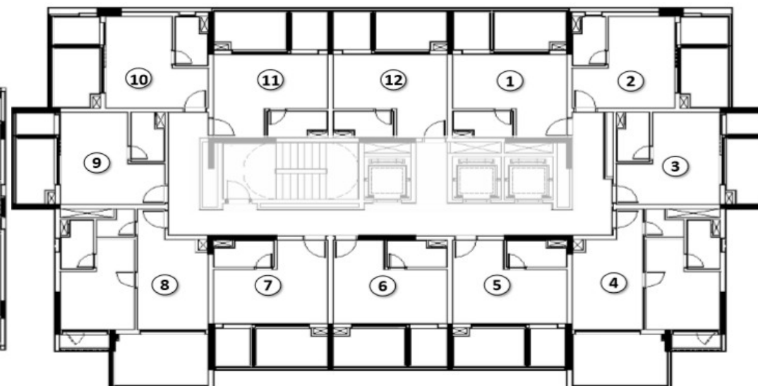
4º AO 24º PAVIMENTO TIPO - RESIDENCIAL
